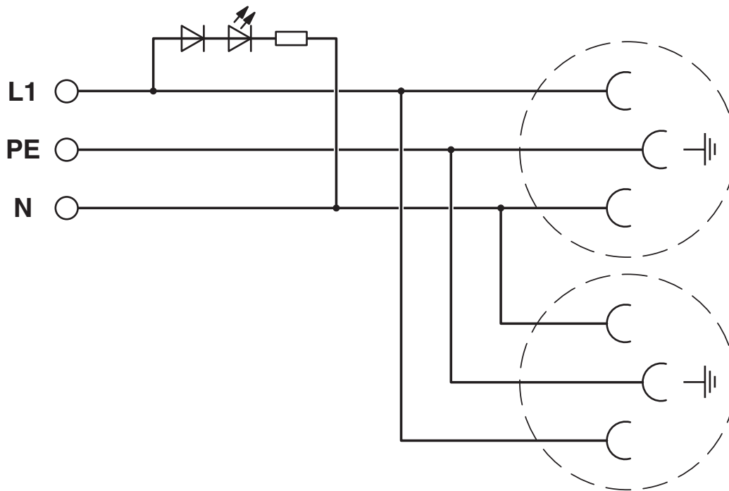
Diagrama eléctrico
