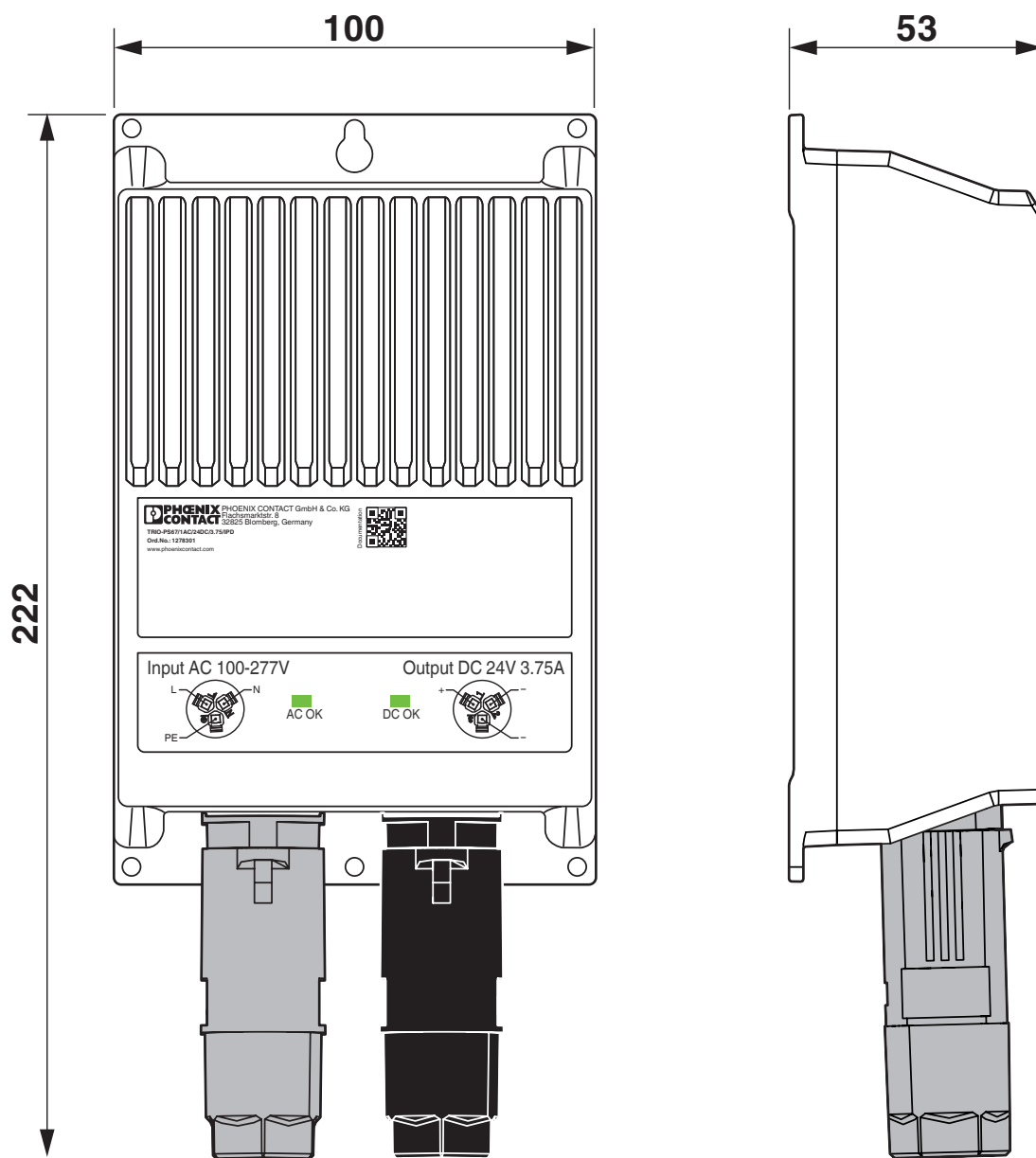
Dimensiones del dispositivo (medidas en mm)
